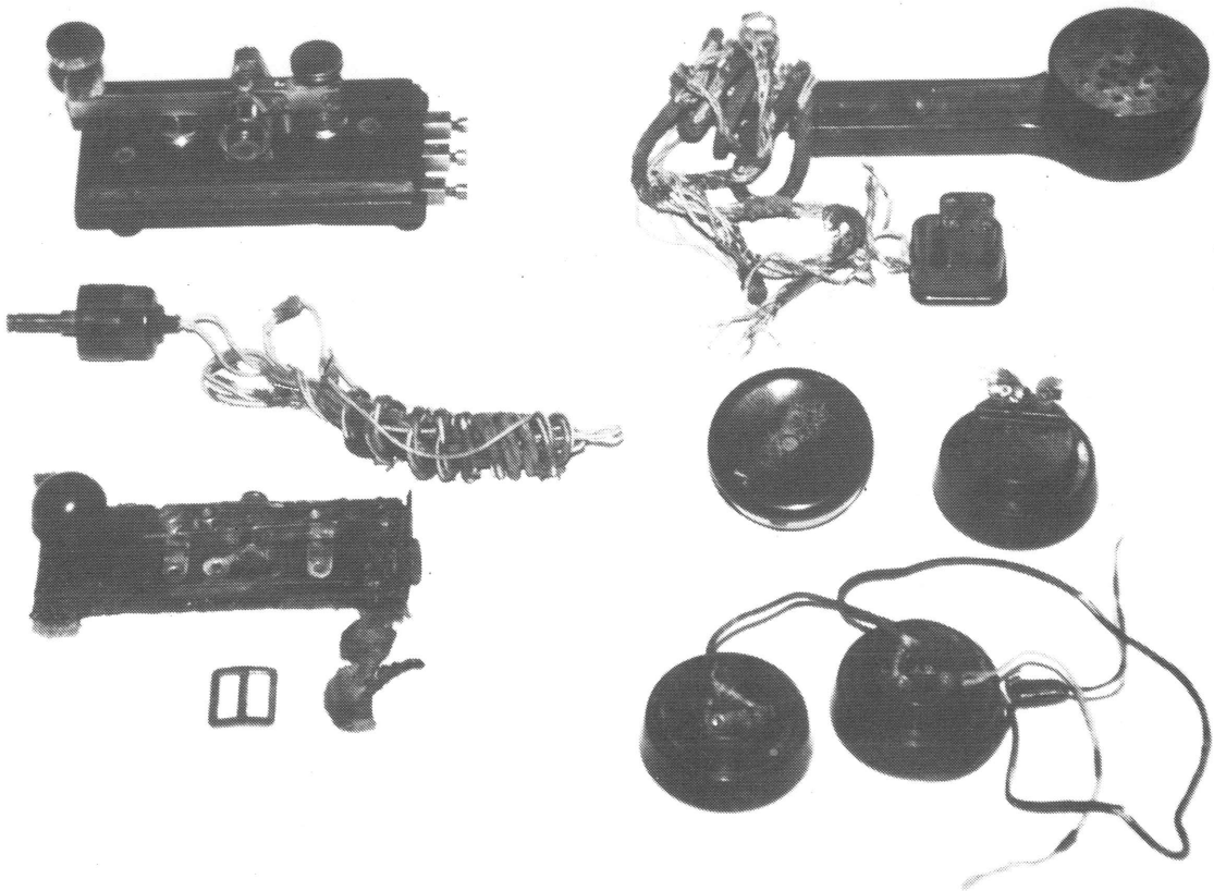
Een deel van de opgegraven onderdelen van de Britse zend-ontvang apparatuur na het schoonmaken. (Foto: B.de Reus).
